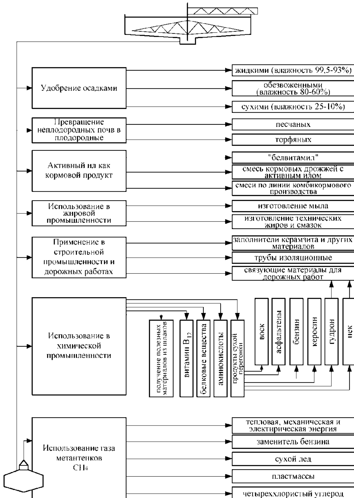
Рисунок 23 – Схема утилизации осадков сточных вод
