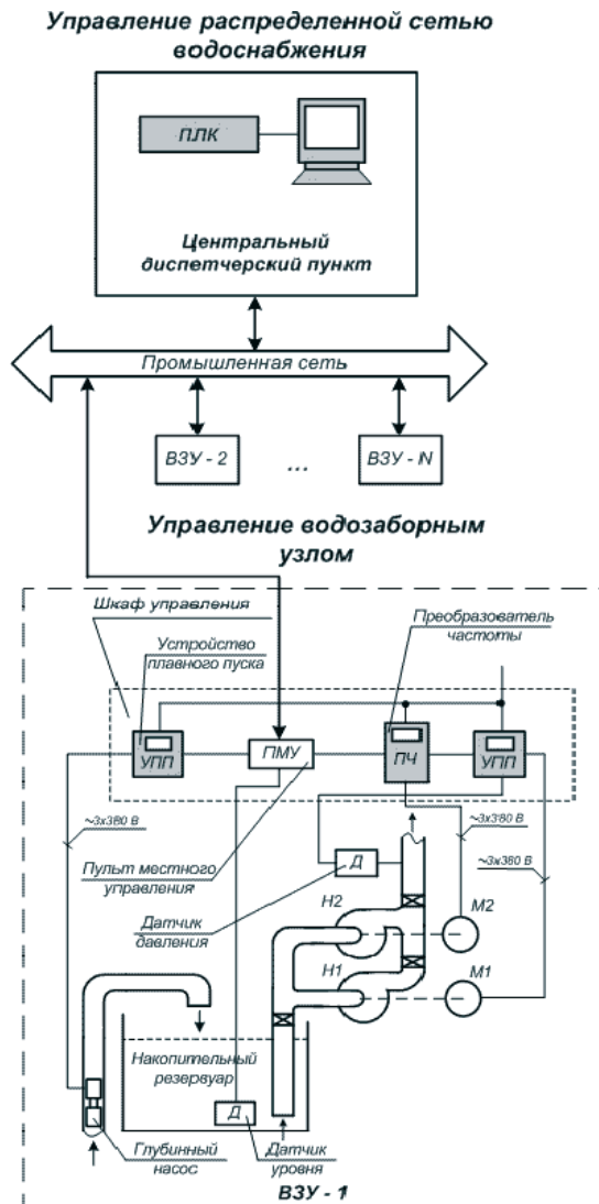
Рисунок 1 - Общая примерная функциональная схема автоматизации ВЗС
