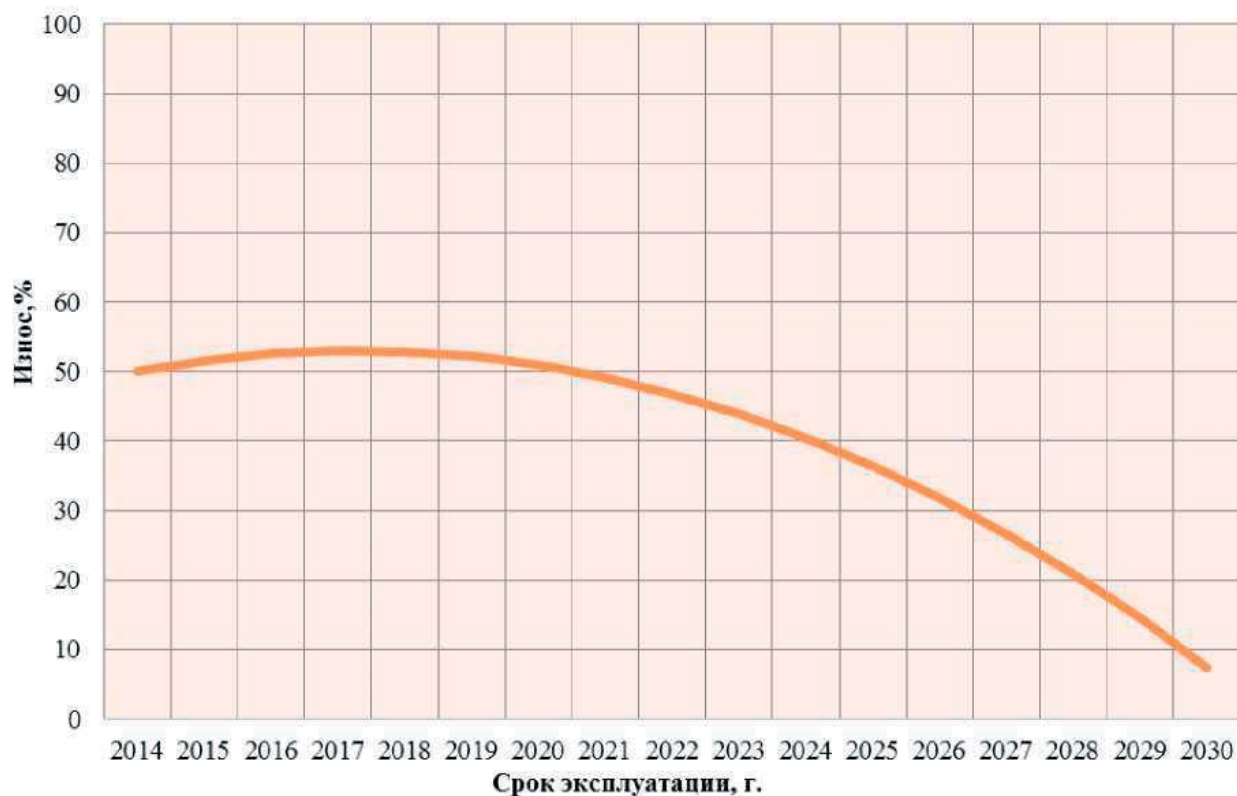
Рис. 7.2.2 - Зависимость износа тепловых сетей от срока эксплуатации
