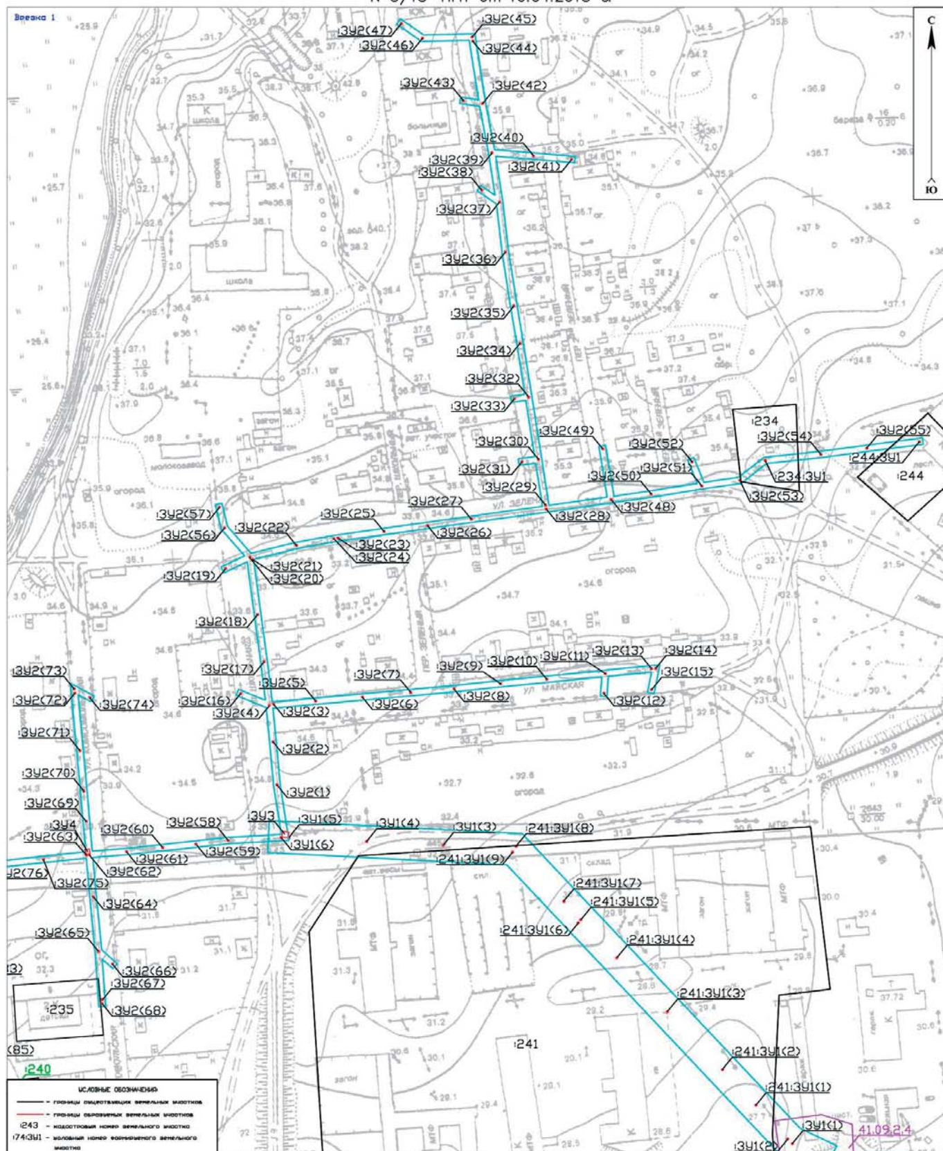
24 Чертеж проекта межевания территории N 3/18-ПМТ от 10.04.2018 г.
